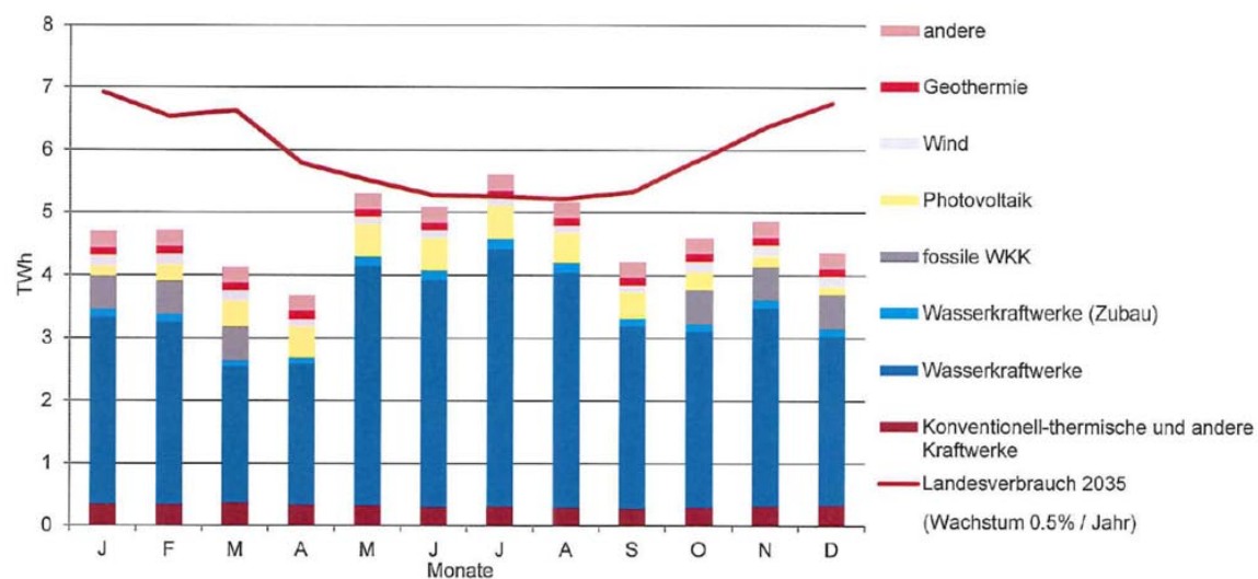
Stromproduktion und Verbrauch Schweiz 2035 ohne Kernkraftwerke und mit Zubau gemäss Energiestrategie 2050
